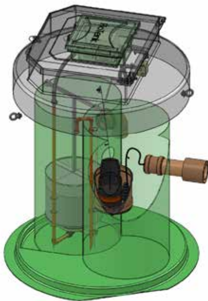
Рис. 1.2 Схема станции FloTenk-BioPurit (принудительная система)
